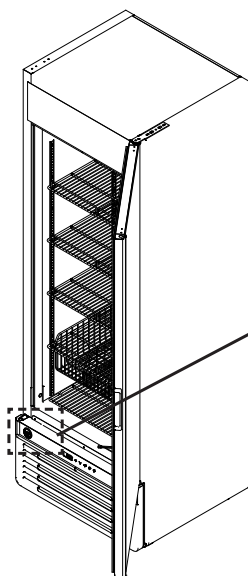
Sauglüfterrad automatisch Schalter (mit Tür geöffnet: Sauglüfterrad getrennt)
